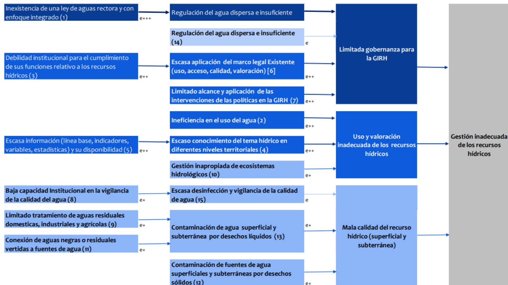
Figura 2. Esquema del modelo explicativo para la gestión de los recursos hídricos
